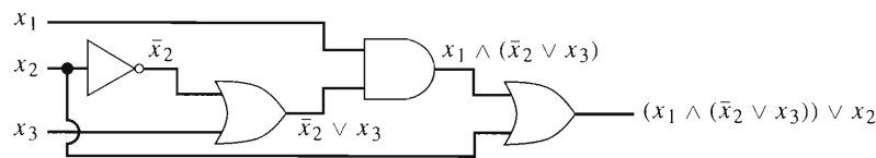
FIGURA 9.1.11 El circuito combinatorio correspondiente a la expresión booleana (x_1 \wedge (\bar{x}_2 \vee x_3)) \vee x_2 .
