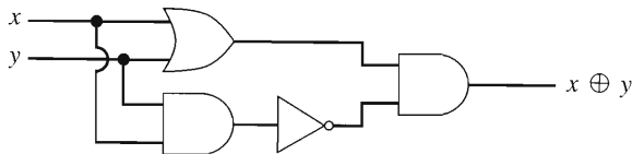
FIGURA 9.5.6 Un circuito combinatorio de cuatro compuertas que calcula el OR exclusivo, x \oplus y , de x y y .
