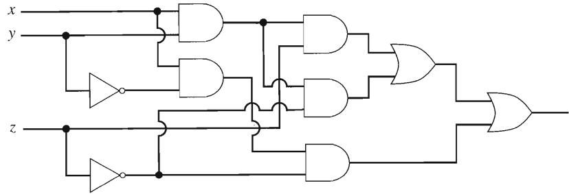
FIGURA 9.5.4 Un circuito combinatorio que calcula f(x, y, z) = xyz \vee xy\bar{z} \vee x\bar{y}\bar{z} .
