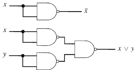
FIGURA 9.5.3 Circuitos combinatorios que sólo utilizan compuertas NAND y calculan \bar{x} y x \vee y . □
