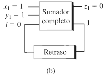
FIGURA 10.1.3 Cálculo de 010 + 011 con el circuito sumador en serie.
