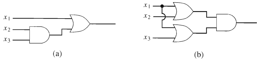
FIGURA 9.2.1 Los circuitos combinatorios (a) y (b) tienen salidas idénticas para entradas idénticas dadas, por lo cual se dice que son equivalentes.
