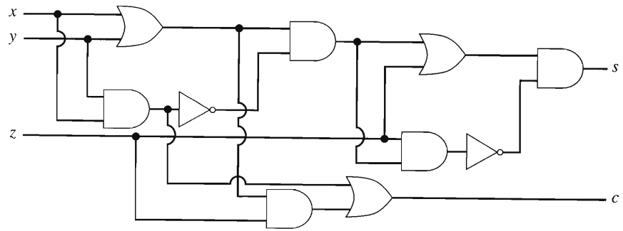
FIGURA 9.5.9 Un circuito sumador completo. □
