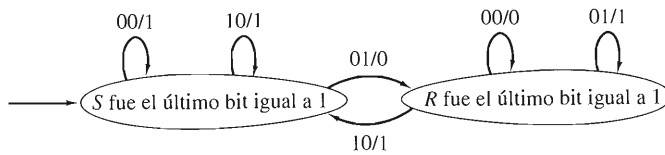
FIGURA 10.1.7 El flip-flop SR como una máquina de estado finito.
