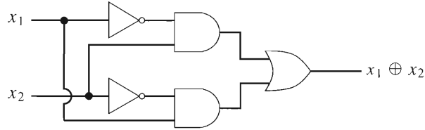
FIGURA 9.4.1 Un circuito combinatorio para el OR exclusivo. □
