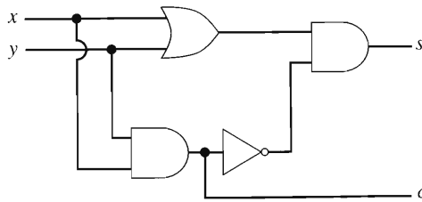
FIGURA 9.5.8 Un circuito semisumador.
