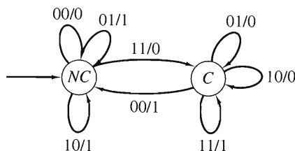
FIGURA 10.1.6 Una máquina de estado finito que realiza la suma en serie.
