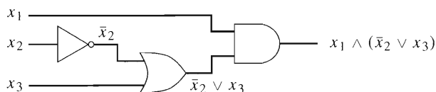
FIGURA 9.1.10 El circuito combinatorio correspondiente a la expresión booleana x_1 \wedge (\bar{x}_2 \vee x_3) .
