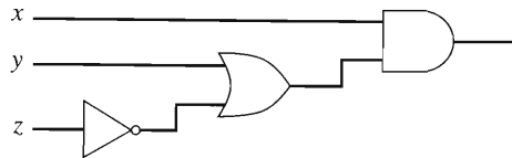
FIGURA 9.5.5 Un circuito combinatorio de tres compuertas, equivalente al de la figura 9.5.4.
