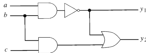
FIGURA 9.5.7 Un circuito combinatorio con dos salidas. □
