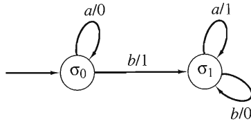
FIGURA 10.1.4 Un diagrama de transición. □
