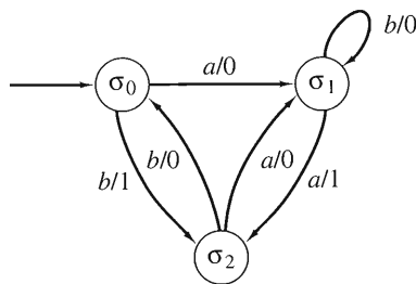
FIGURA 10.2.4 El autómata de estado finito de la figura 10.2.3, ahora como un diagrama de transición de una máquina de estado finito.
