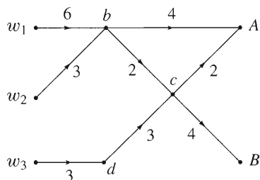
FIGURA 8.1.3 Una red de bombeo. El agua de las ciudades A y B se obtiene de los pozos w_1 , w_2 y w_3 . Las capacidades aparecen sobre las aristas.
