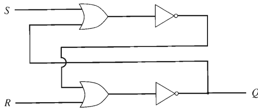
FIGURA 10.1.8 Una implantación del flip-flop SR mediante un circuito secuencial. \square
