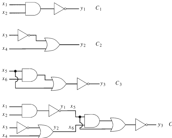
FIGURA 9.1.7 El circuito combinatorio C se obtiene conectando los circuitos combinatorios C_1 , C_2 y C_3 . □
