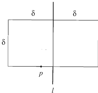
FIGURA 11.1.2
