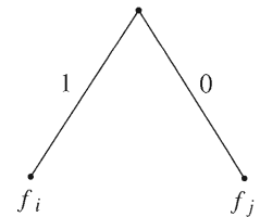
FIGURA 7.1.10
