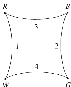
FIGURA 6.8.9
