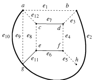
FIGURA 7.3.1
