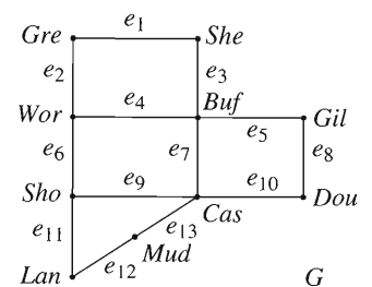
FIGURA 6.1.2
