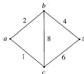
FIGURA 7.4.4
