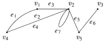
FIGURA 6.5.4
