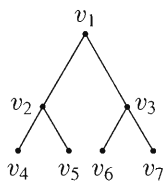
FIGURA 7.1.4
