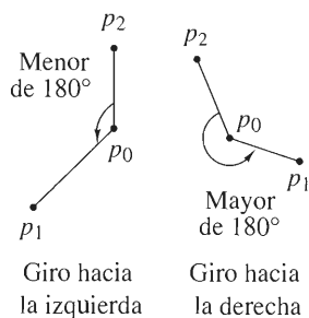
FIGURA 11.3.5
