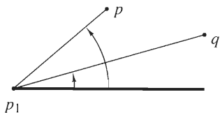
FIGURA 11.3.7
