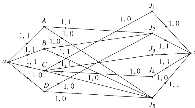
FIGURA 8.4.3 El problema de acoplamiento (figura 8.4.1) como una red de acoplamiento. □
