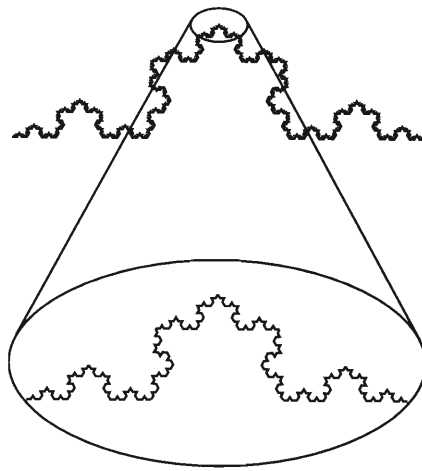
FIGURA 10.3.2 La naturaleza fractal del copo de nieve de von Koch. Cuando la parte superior del copo de nieve de von Koch se extrae y se amplía, se asemeja a la curva original.
