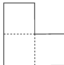
FIGURA 1.6.3 Un triominó.
