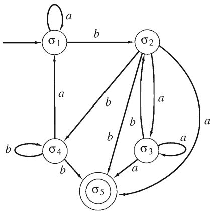
FIGURA 10.5.8 Un autómata de estado finito no determinista con un estado de aceptación equivalente al autómata de estado finito de la figura 10.5.7.
