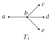
FIGURA 7.8.1 Un árbol.
