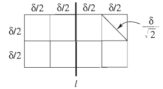
FIGURA 11.1.3
