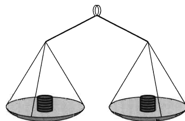
FIGURA 7.7.2 Una balanza de platillos para comparar pesos de monedas.
