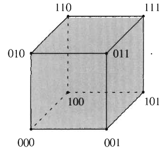
FIGURA 6.1.9 El 3-cubo.
