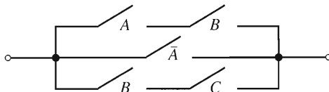
FIGURA 9.1.12 Un circuito de conmutación.
