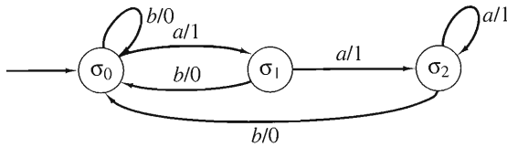
FIGURA 10.2.1 El diagrama de transición para el ejemplo 10.2.2. □
