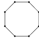
FIGURA 6.3.9
