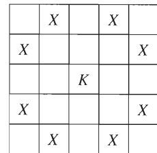
FIGURA 6.3.10
