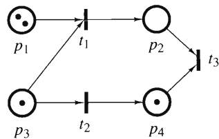
FIGURA 8.5.3 Una red de Petri marcada. □
