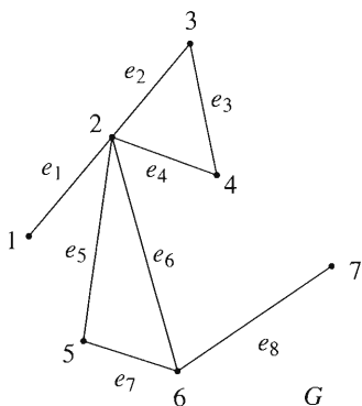
FIGURA 6.2.1
