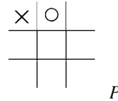
FIGURA 7.9.5
