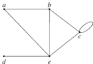
FIGURA 6.5.1
