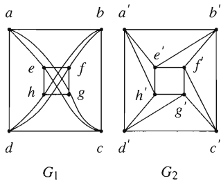
FIGURA 6.6.5
