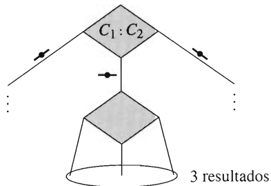
FIGURA 7.7.6 Un algoritmo para el juego de cuatro monedas que comienza comparando una moneda con otra.
