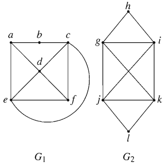
FIGURA 6.6.4
