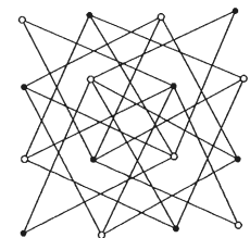
FIGURA 6.3.11
