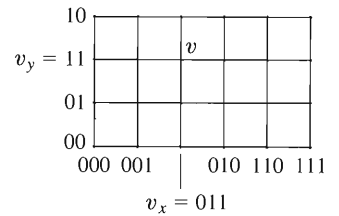
FIGURA 6.6.2
