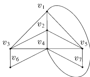
FIGURA 6.2.10
