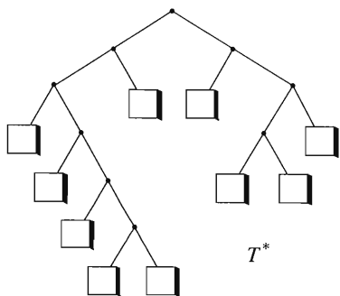
FIGURA 7.5.6
