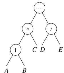
FIGURA 7.6.7 La representación mediante un árbol binario de la expresión (A + B) * C - D/E .
