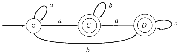
FIGURA 10.4.3 El diagrama de transición del autómata de estado finito no determinista del ejemplo 10.4.6. □
