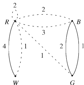
FIGURA 6.8.7
