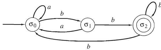
FIGURA 10.2.5 El diagrama de transición para el ejemplo 10.2.4. □
