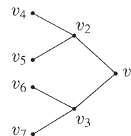
FIGURA 7.1.2
