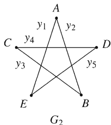
FIGURA 6.6.1 Gráficas isomorfas.
