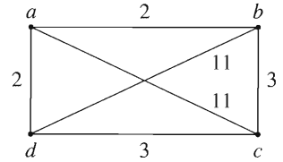
FIGURA 6.3.8
