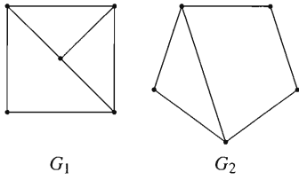
FIGURA 6.6.3
