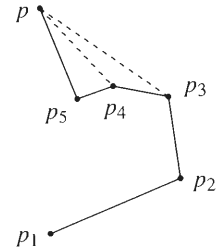
FIGURA 11.3.9
