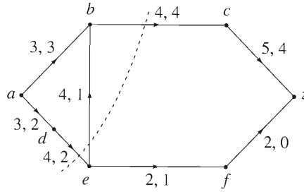
FIGURA 8.3.1 Un corte en una red. La línea punteada divide los vértices en los conjuntos P = \{a, b, d\} y \bar{P} = \{c, e, f, z\} produciendo el corte (P, \bar{P}) . □
