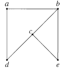
FIGURA 6.5.2
