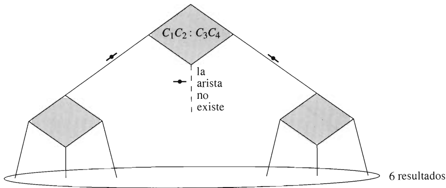
FIGURA 7.7.5 Un algoritmo para el juego de cuatro monedas que comienza comparando dos monedas con dos monedas.
