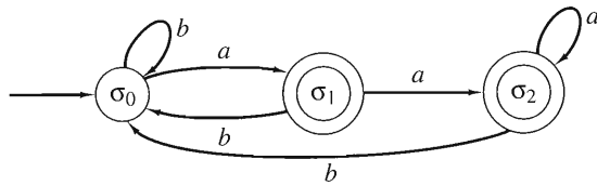
FIGURA 10.2.2 El diagrama de transición de la figura 10.2.1, con los estados de aceptación encerrados en círculos dobles y omitiendo los símbolos de salida.
