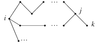
FIGURA 6.5.3
