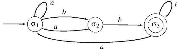
FIGURA 10.5.4 El autómata de estado finito del ejemplo 10.5.7, que acepta a L .
