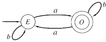
FIGURA 10.2.7
