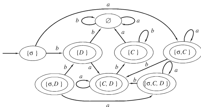
FIGURA 10.5.3 Un autómata de estado finito equivalente al autómata de estado finito no determinista de la figura 10.4.6. \square
