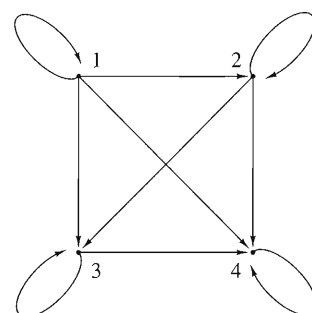
FIGURA 2.4.1
