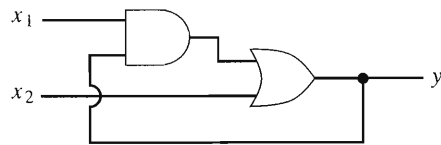
FIGURA 9.1.6 Un circuito que no es un circuito combinatorio. □
