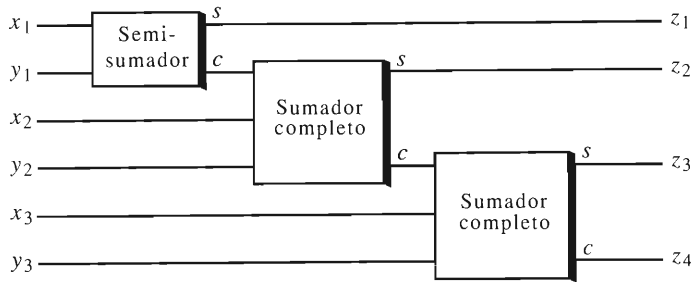
FIGURA 9.5.10 Un circuito combinatorio que calcula la suma de dos números de tres bits cada uno.
